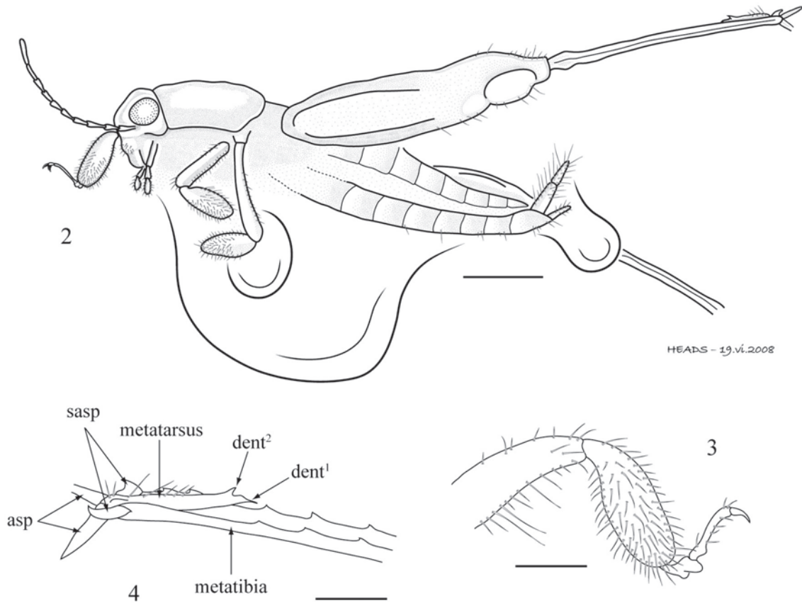
Figs 2-4: Burmadactylus grimaldii gen. et sp.nov. (AMNH Bu1452).
